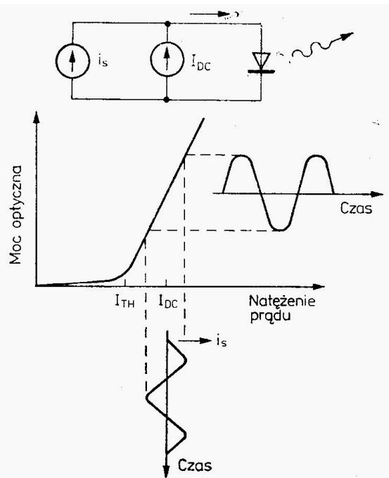
Rys. 6.24. Modulacja analogowa w diodzie laserowej
