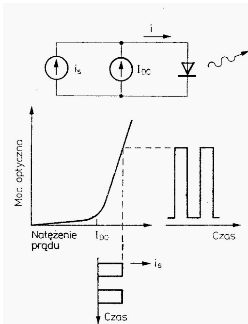
Rys. 6.23. Modulacja cyfrowa w diodzie laserowej
